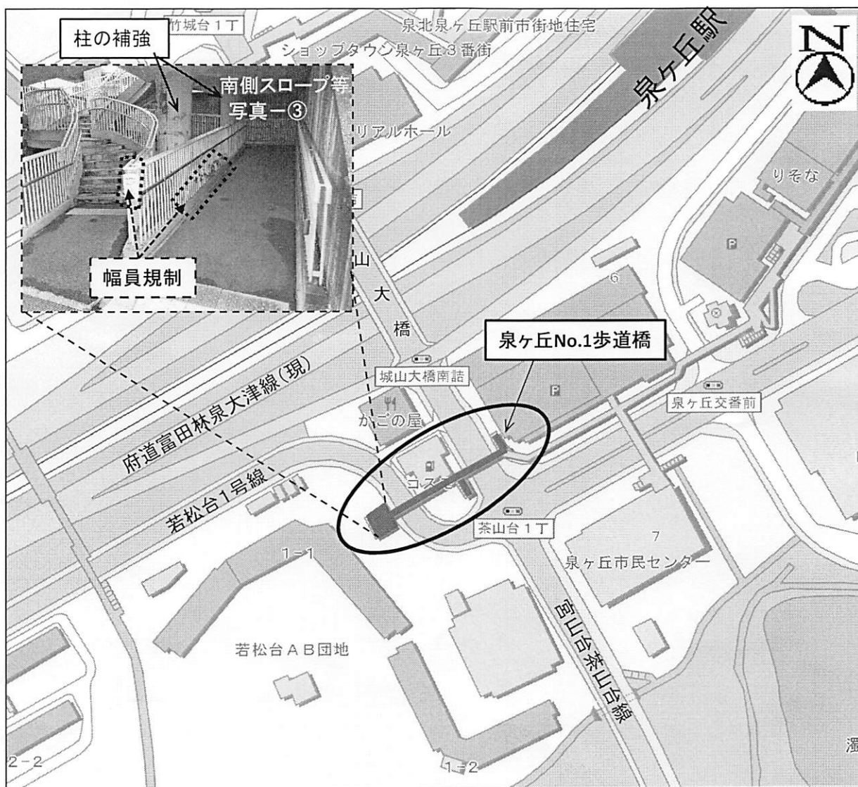
泉ヶ丘No. 1歩道橋現況写真
